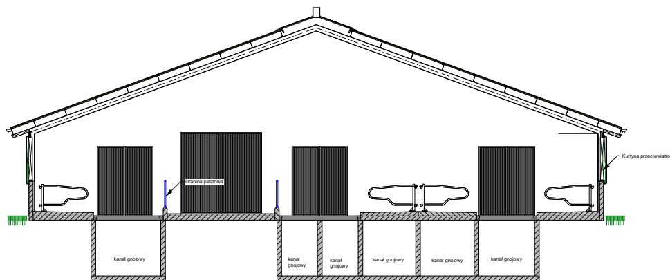
Przekrój A-A
