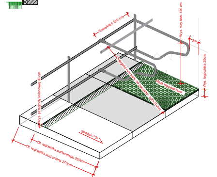
Schemat legowiska
